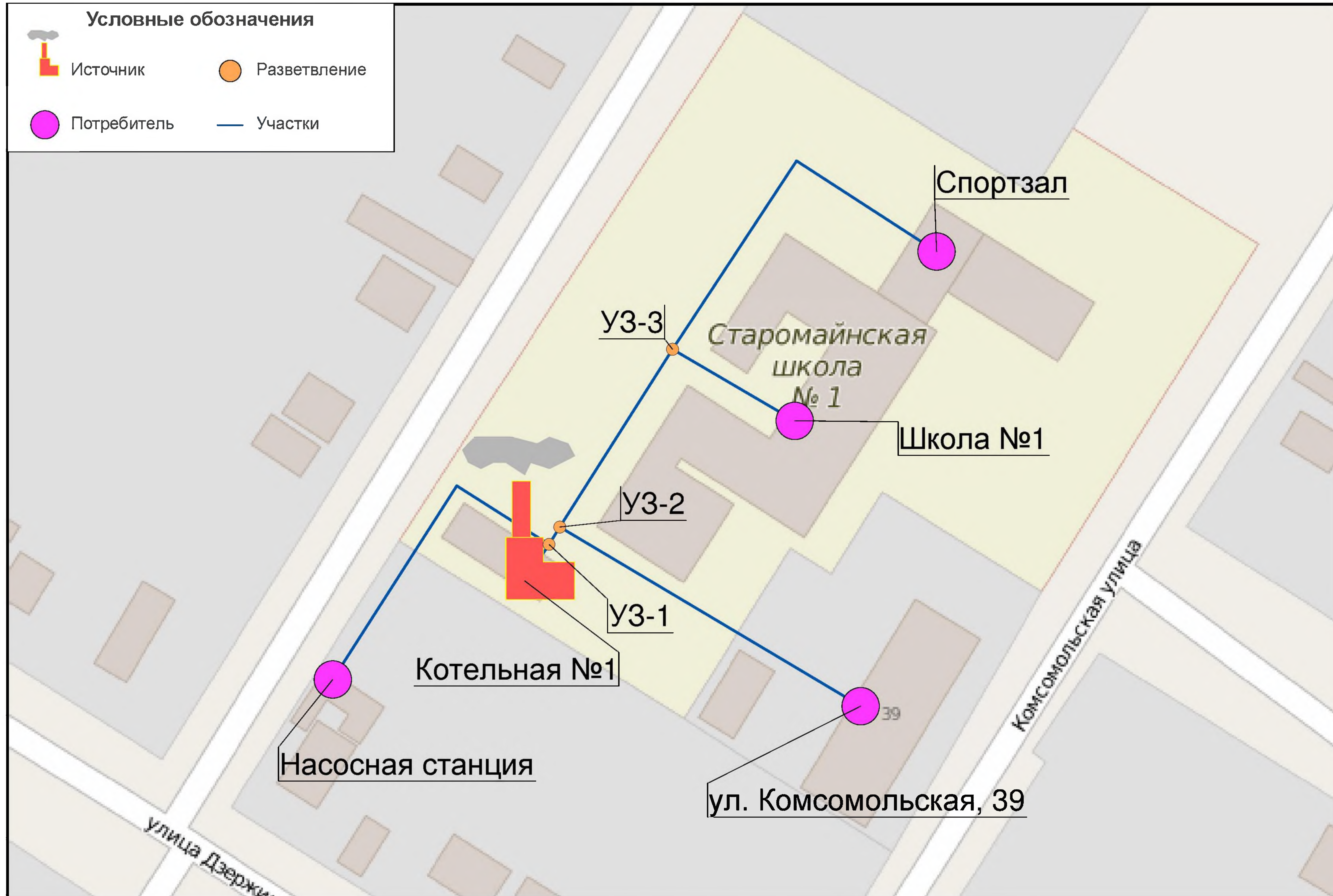
Схема тепловых сетей котельной №1 (школа)
