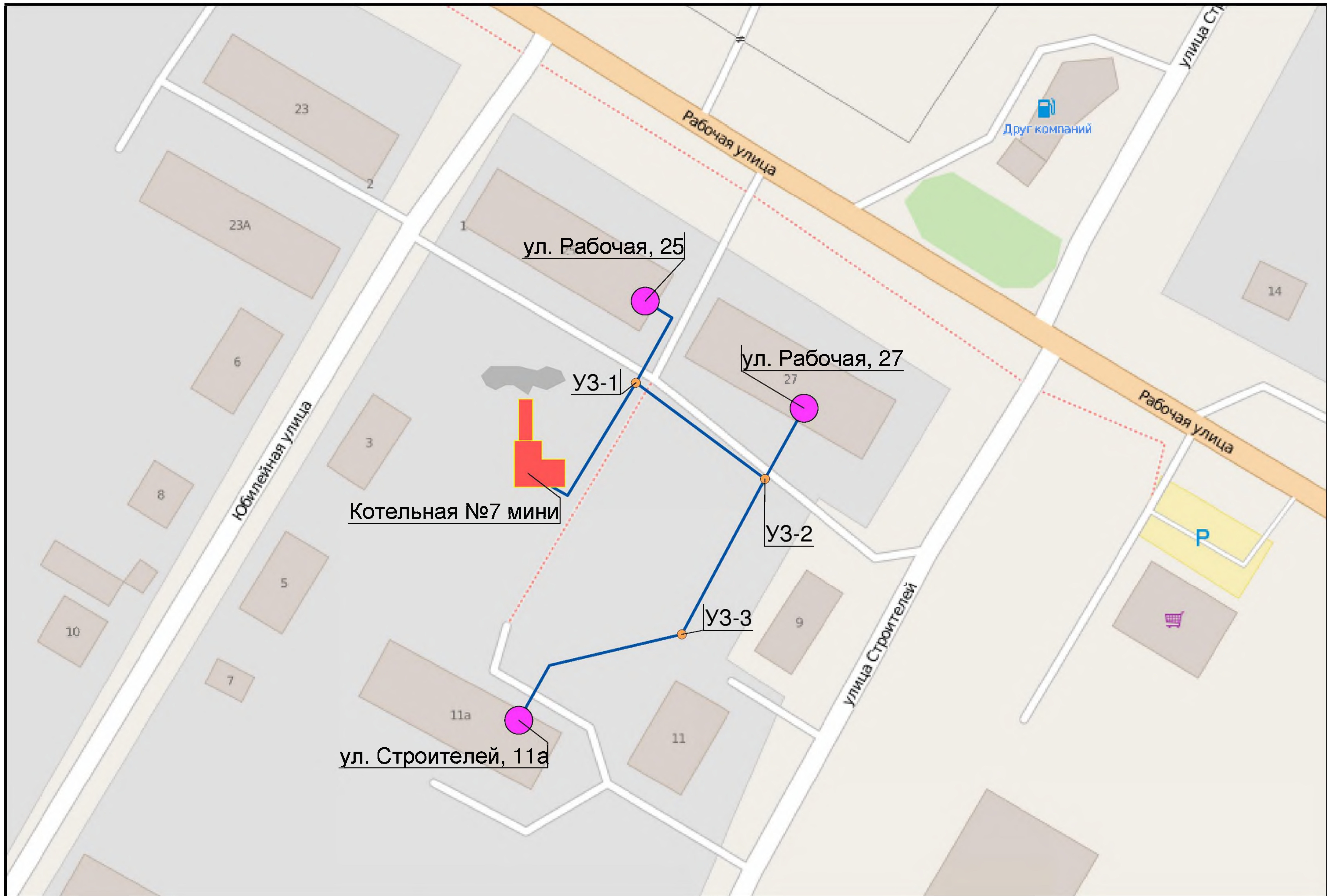
Схема тепловых сетей котельной №7 мини
