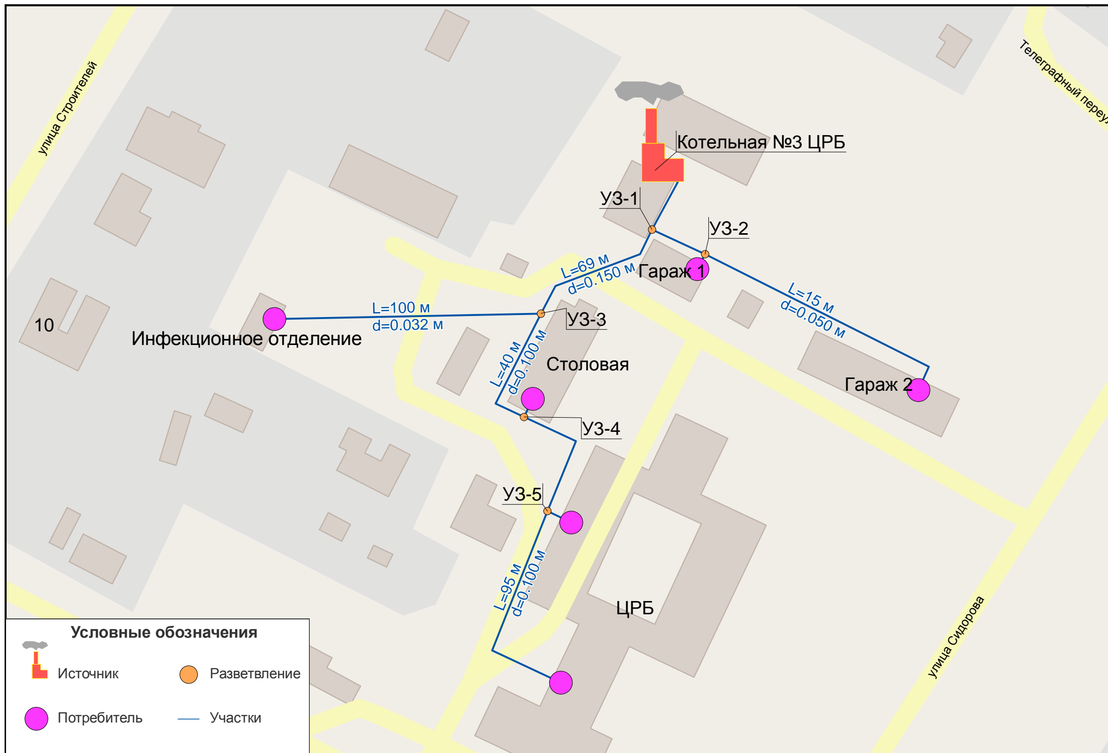
Рис. 3. Схема тепловых сетей котельной №3 "ЦРБ"
